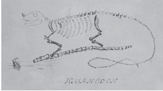
شكل ١-٦: رسم مانتل التخطيطي الذي يعيد فيه بناء شكل الإجواندون (١٨٣٤ تقريباً).
