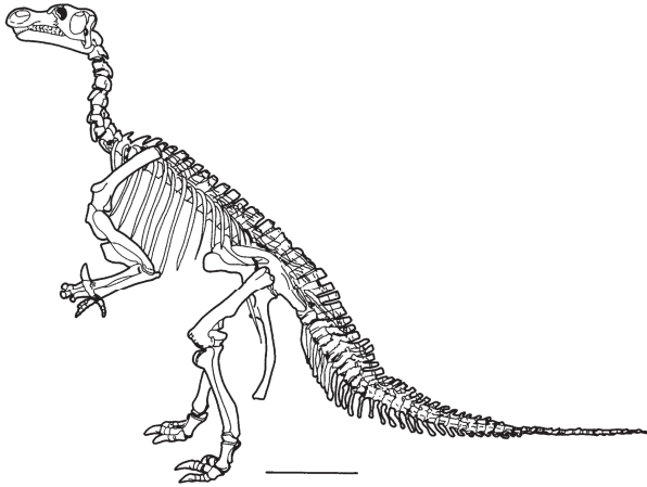
شكل ١-٩: رسم لهيكل عظمي يخص ديناصور الإجانودون.
