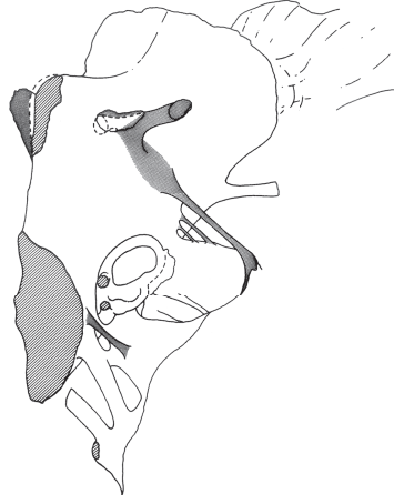
شكل ٣-٨: (جهة اليسار): صورة مائلة للقالب الطبيعي المصنوع من تجويف مخ الإيواندون. (جهة اليمين): رسم تخطيطي لتجويف المخ يوضح تكوين الأذن، والأعصاب، والأوعية الدموية، وفصوص الشم.
