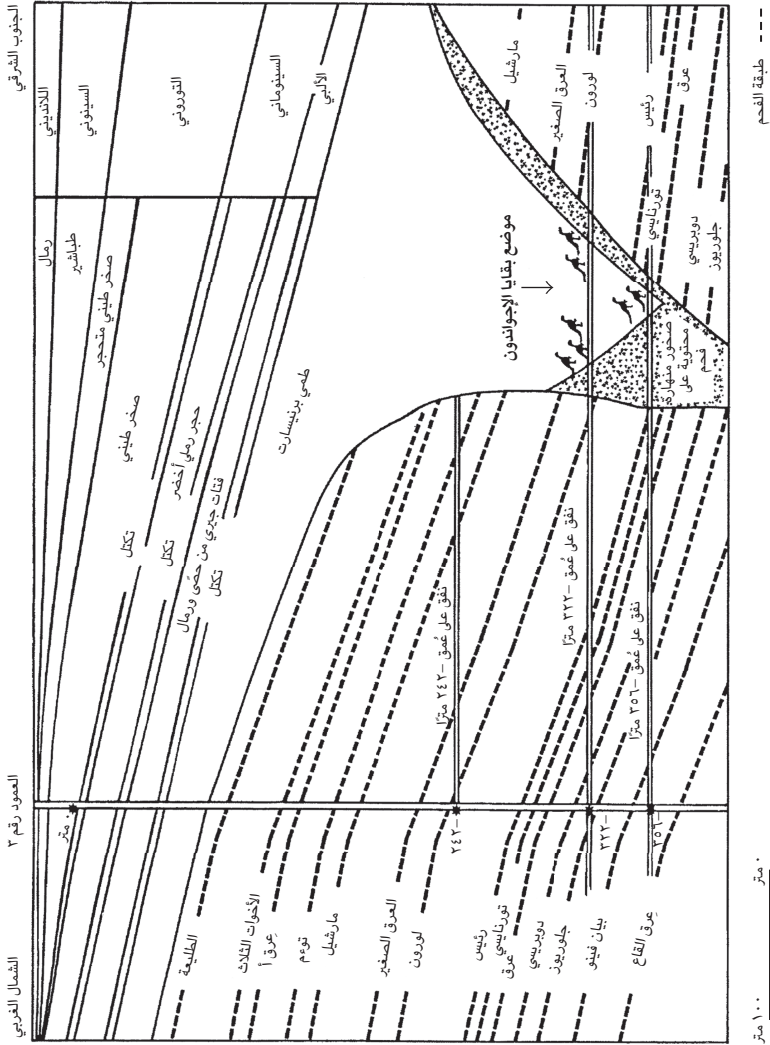
شكل ١-٢: مقطع جيولوجي لمنجم برنيسارت.
