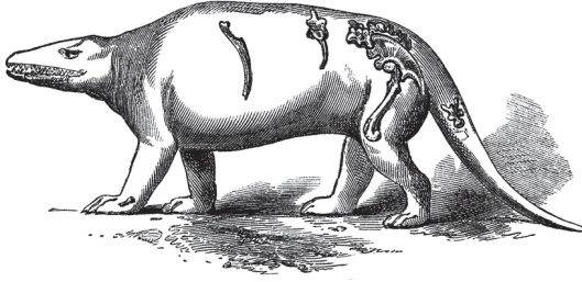
شكل ١-٧: نموذج أُعيدَ بناؤه لديناصور الميجالوصور لأوين (١٨٥٤ تقريبًا).
