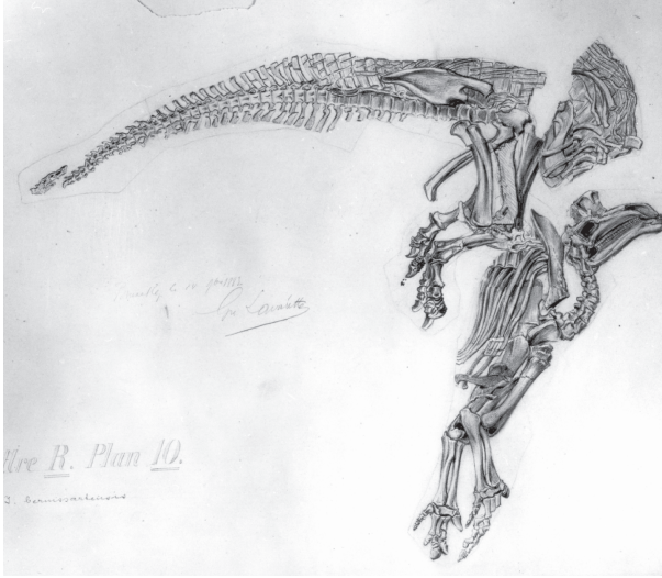
شكل ٣-٣: رسم لافاليت لهيكل الإخواندون الموجود في الشكل ٣-٢.
