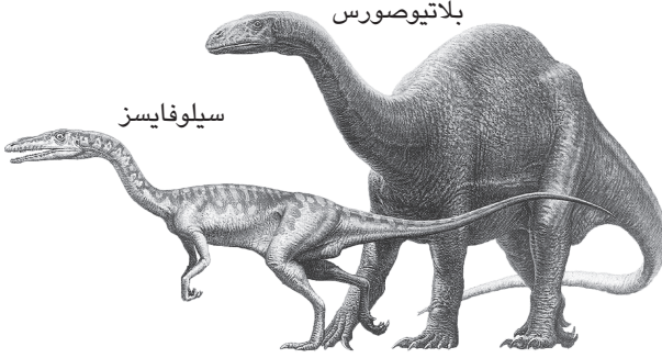
شكل ٤-٣: سحليات الورك من العصر الترياسي. الديناصور سيلوفائيسز من الثيروبودات الأولى، والديناصور بلاتيوصورس من الصوربودات.
