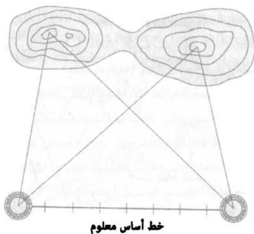
الشكل (46): تحديد موقع قمتي جبلين باستخدام المثلثات من نقاط تحكّم على خط أساس معروف.
