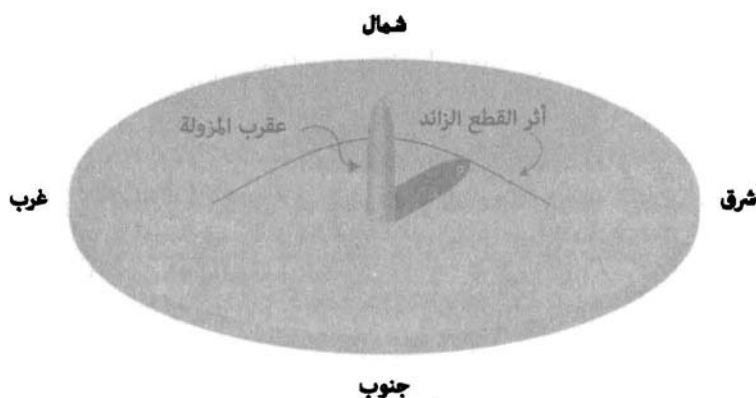
الشكل (81): مبدأ البوصلة الشمسية. يظهر هذا المثال الظل في وقت ما في فترة بعد الظهر خلال الصيف في نصف الكرة الشمالي.
