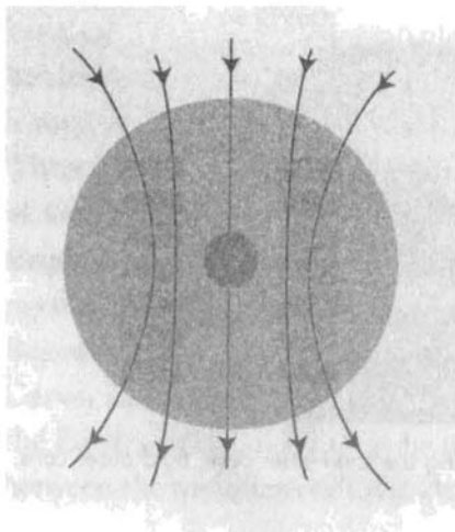
الشكل (43): تؤدي حركية جريان السائل في النواة الخارجية إلى نشوء تأثير يدعم نفسه ذاتيا يولد الحقل المغناطيسي الأرضي.
